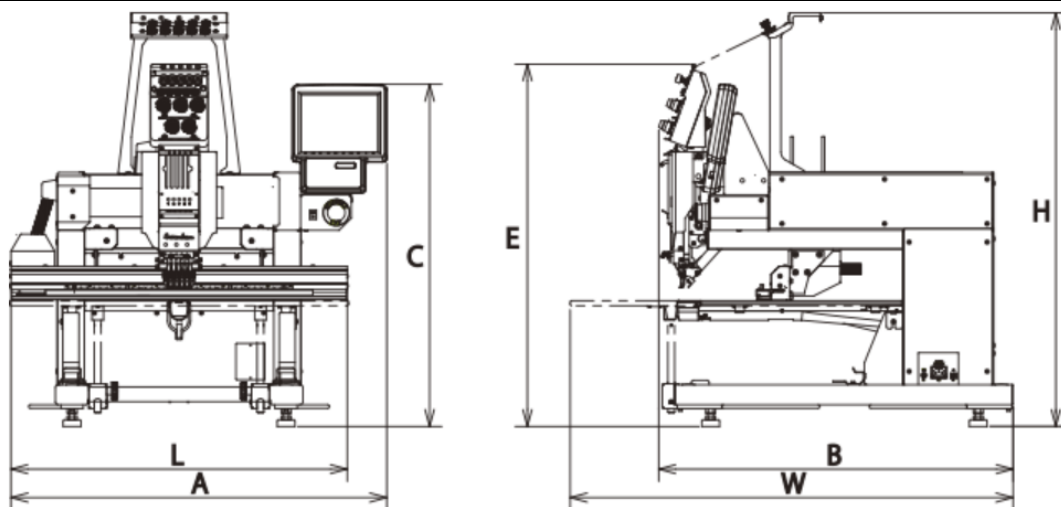
MODEL BEKT-S501CBⅢ
